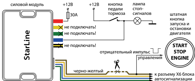
Схема 2: слаботочное управление кнопкой «старт-стоп»
