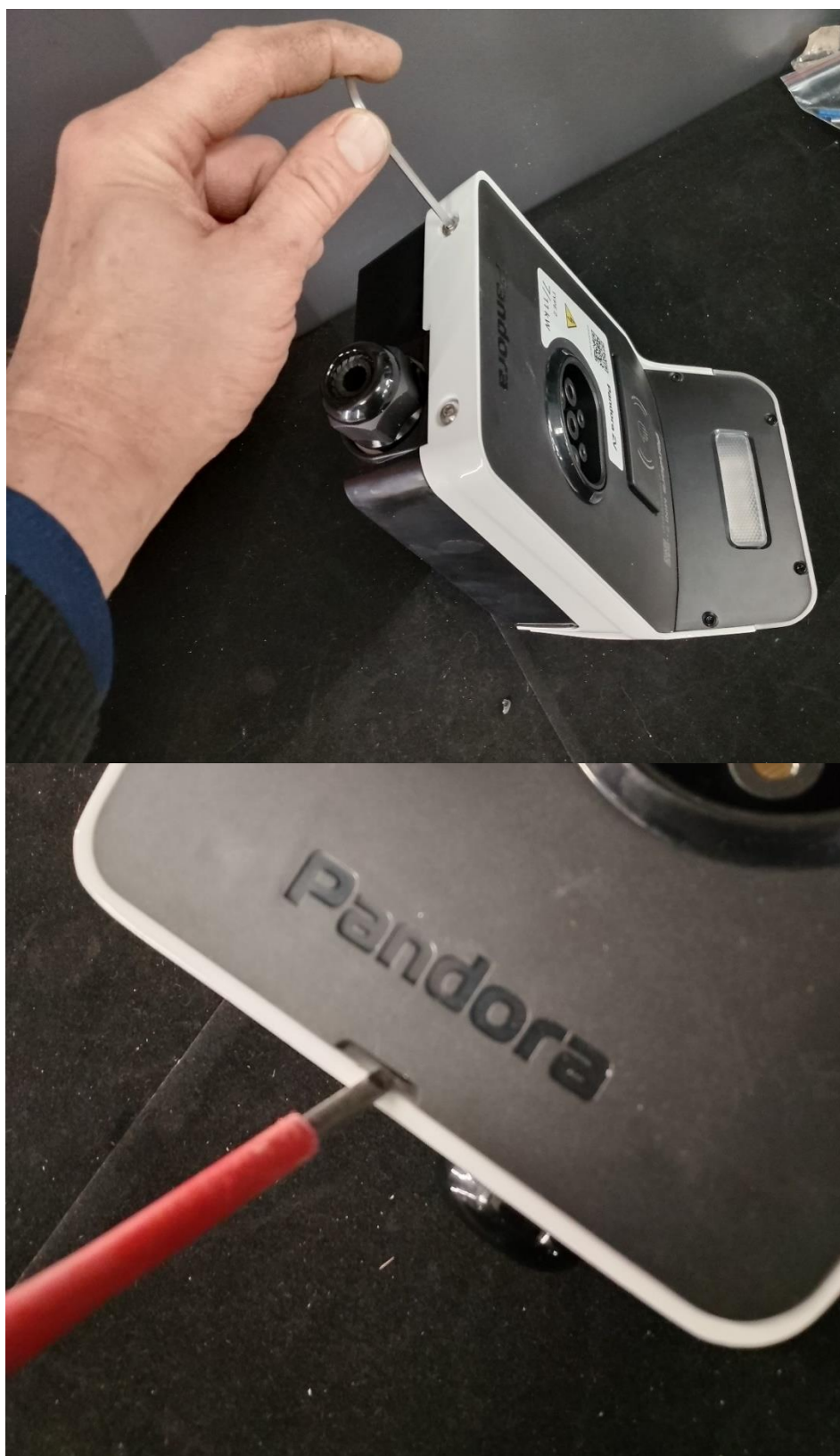
Рисунок 2. Снятие лицевой панели станции
