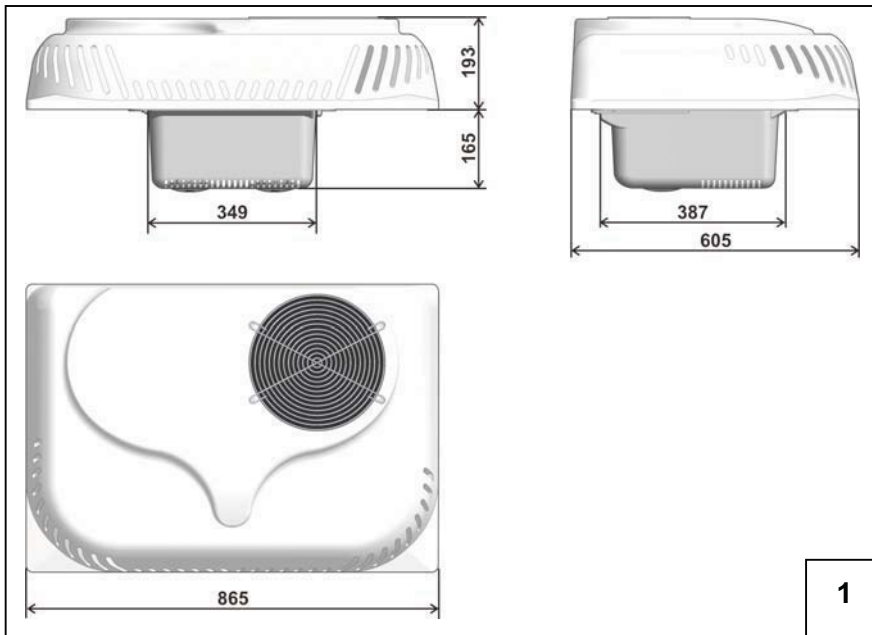
Основные размеры
